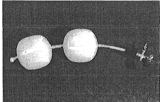
Kettős ballon DN200 egyedi ballon felfújással
